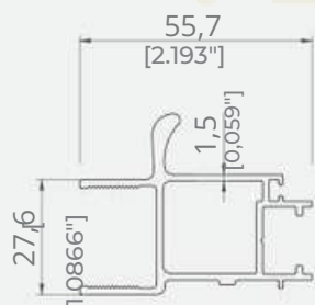
PROFIL CAPAC STICLĂ 60X17,2
